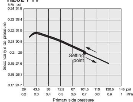
RZ32-F11
