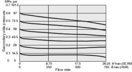
RZ32-F11-02
