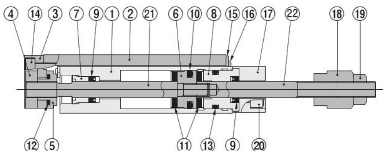
MGAP□12, 16, 20
